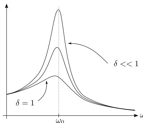
Abbildung 5.2: Resonanzamplitude R
